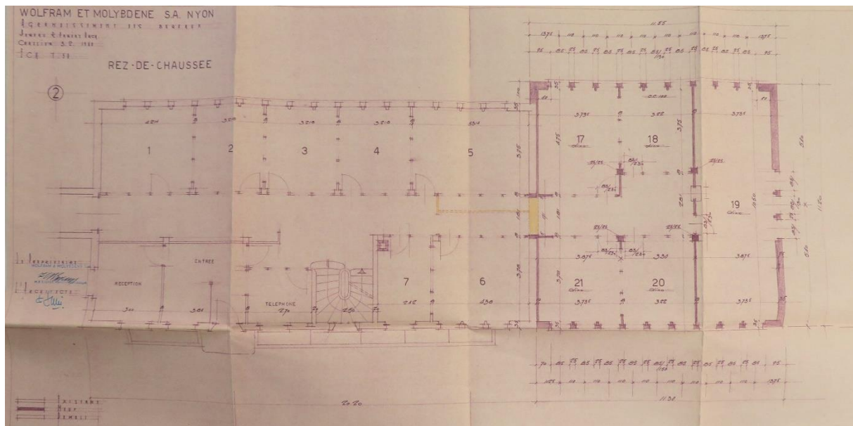
Fig. 11. Agrandissement du bâtiment administratif, plan du rez-de-chaussée, 1960, par Roger Paréaz arch. pour Wolfran et Molybdène SA (Archives communales de Nyon, police des constructions, dossier 2086). La partie de gauche, pour laquelle il n'existe pas d'archives, a été construite en 1957.
