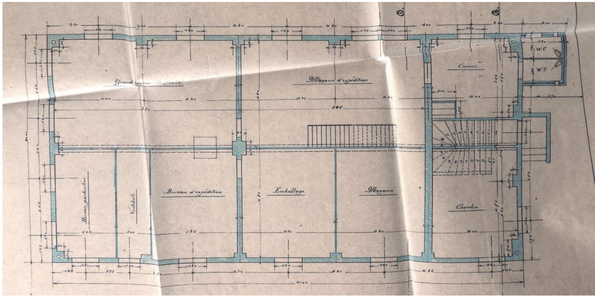
Fig. 4. Plan du rez-de-chaussée, A. Jonneret-Canel ing., novembre 1902 (Archives communales de Nyon, police des constructions, dossier K-305.25).
