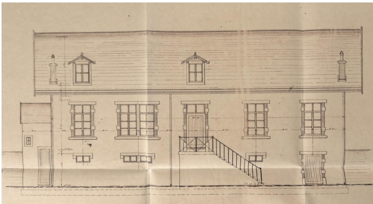
Fig. 5. Elévation ouest, A. Jonneret-Canel ing., novembre 1902 (Archives communales de Nyon, police des constructions, dossier K-305.25).
