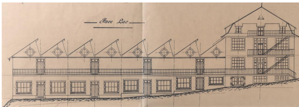
Fig. 8. Elévation sud, A. Jonneret-Canel ing., novembre 1906 (Archives communales de Nyon, police des constructions, dossier K-308.24).
