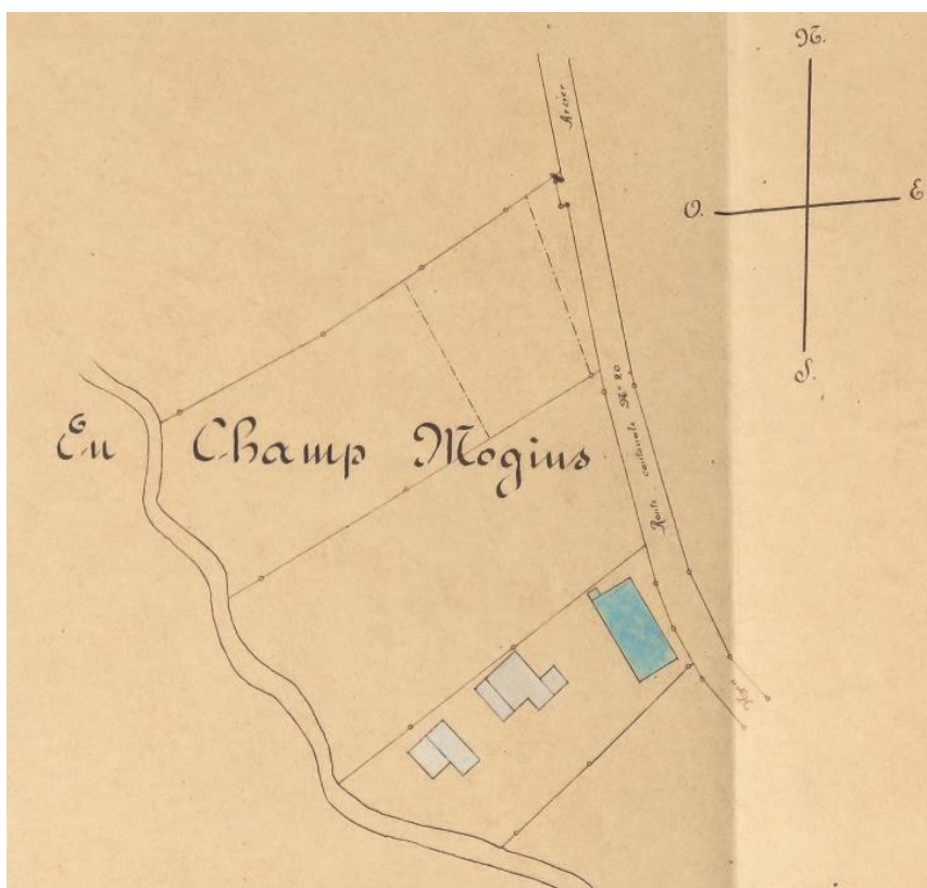
Fig. 3. Plan de situation, A. Jonneret-Canel ing., novembre 1902 (Archives communales de Nyon, police des constructions, dossier K-305.25). En bleu, le nouveau bâtiment s'ajoutant aux deux autres déjà occupés par Th. Mühlethaler.
