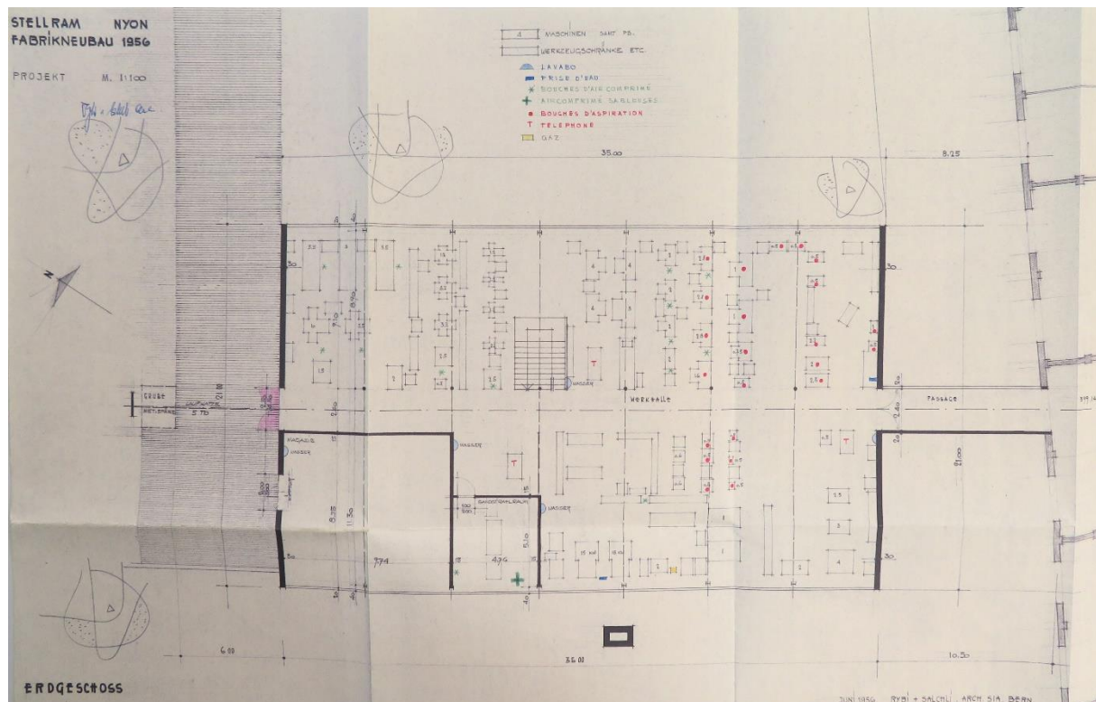
Fig. 13. Projet de fabrique Stellram, plan du rez-de-chaussée, 1956, Rybi et Salchi arch. pour Wolfram et Molybdène (Archives communales de Nyon, police des constructions, dossier 1785).
